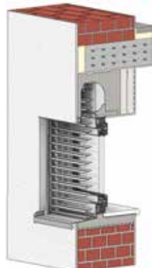
Monolithisch mit Rollladenkastensystem RA-RS
