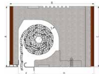
Revision Außen MS42 beidseitig
